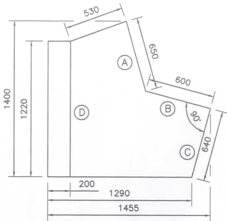
END ELEVATION
